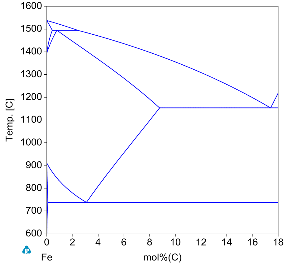
Fe-C 2元系状態図 Graphite基準
